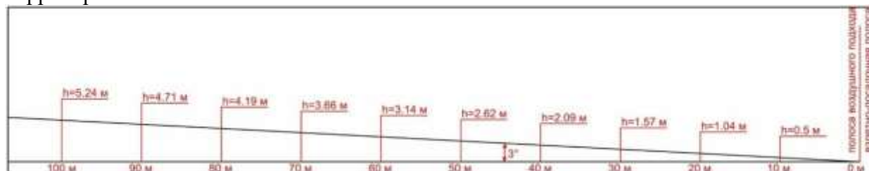
Рисунок 1. Ограничения по высоте застройки на различном удалении от торца взлетно-посадочной полосы (на расстоянии от 0 до 100м)
